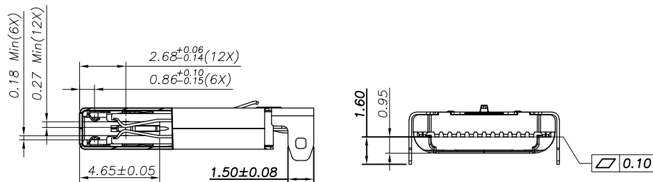
SECTION:A-A SCALE 1:1
