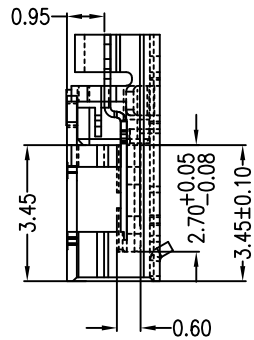
SEC A-A
