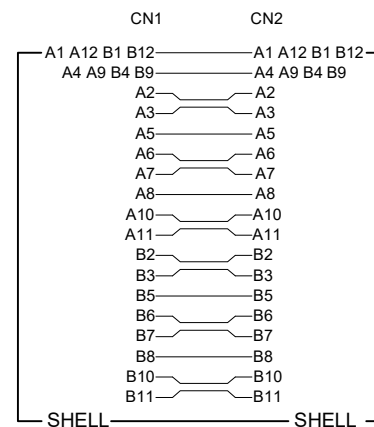
接点表
