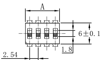
Dimensions (unit:mm)
