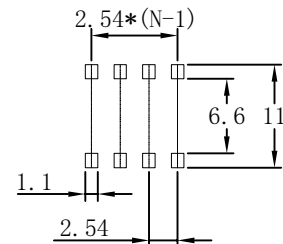
P.C.B.Layout(unit:mm)
