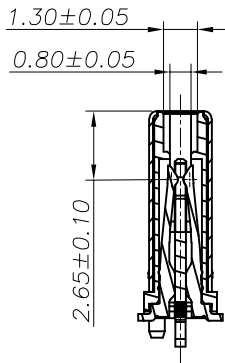
SECTION:B-B
