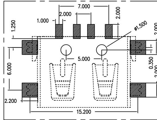
PCB参考图
