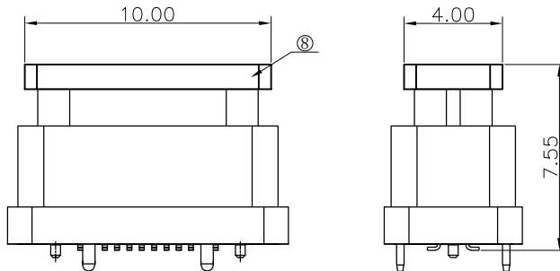
CAP尺寸图
