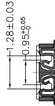
SEC A-A
